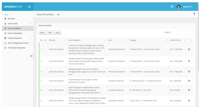
Gambar 18. Halaman Penelitian Pada User Kaprodi
