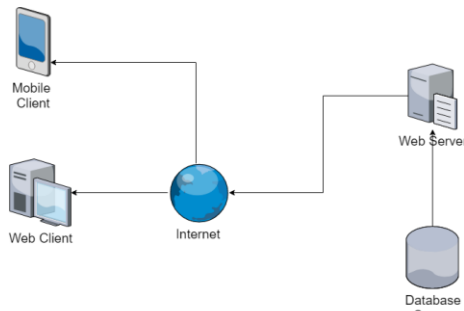
Gambar 3. Arsitektur Aplikasi
